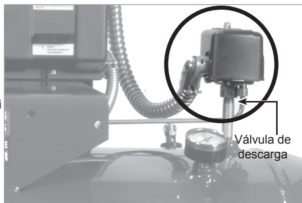
Figura 9 - Presostato
